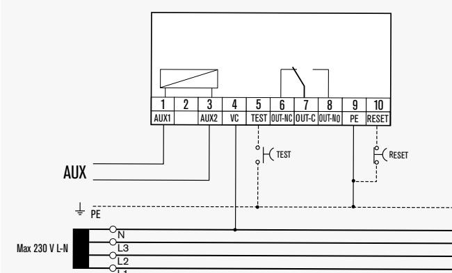
RI-R22 - Schema Elettrico
