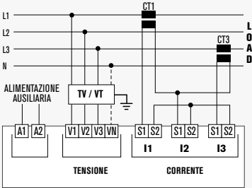
TRIFASE CON INSERZIONE ARON MEDIANTE TV
