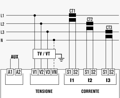
TRIFASE CON E SENZA NEUTRO MEDIANTE TV
