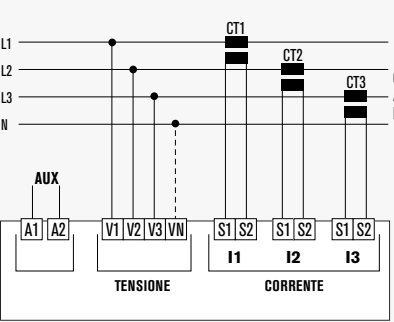
TRIFASE CON E SENZA NEUTRO
