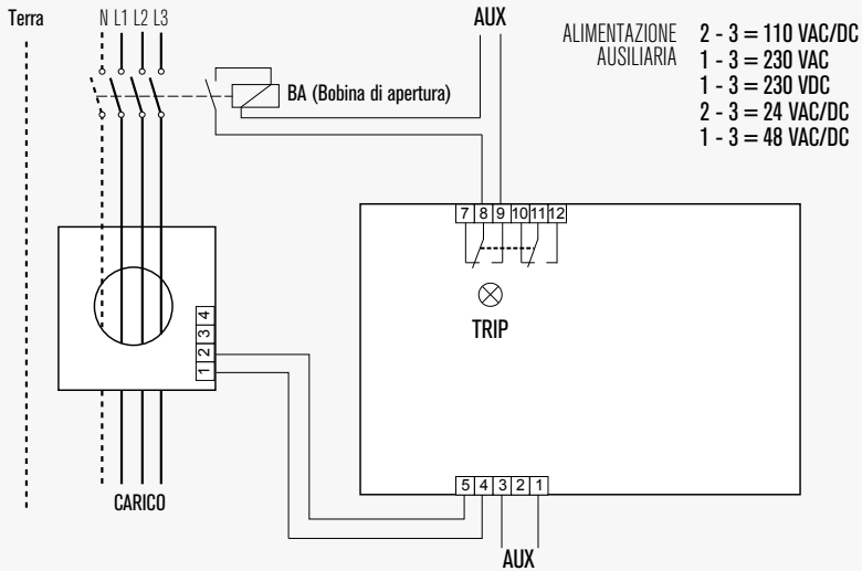
ELR-7 - Schema Elettrico
