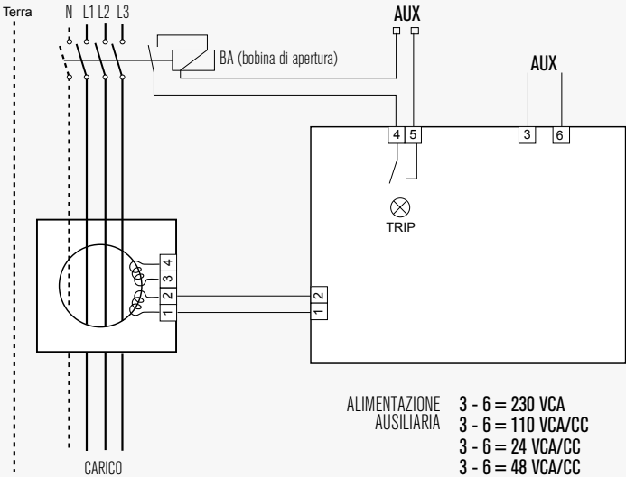
ELR-1D - Schema Elettrico
