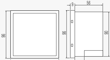
RDU - Dimensioni (mm)
