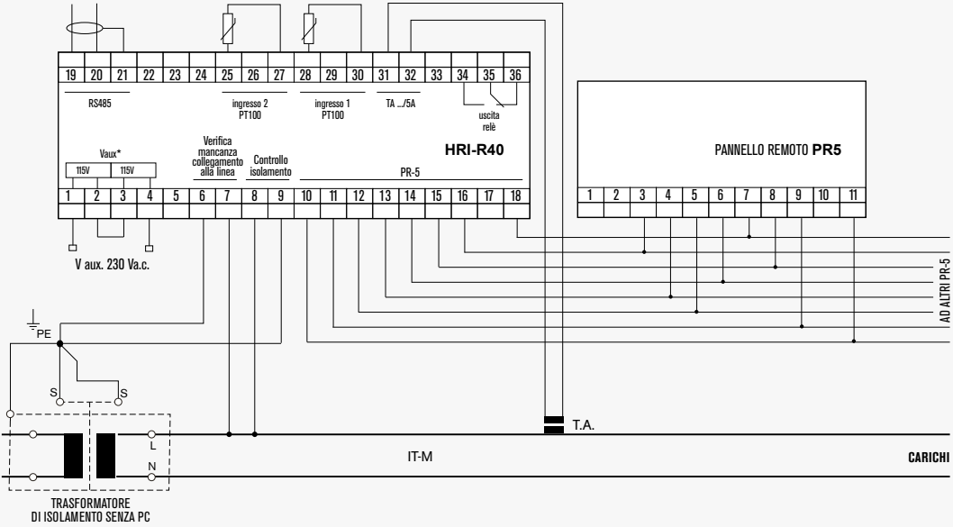
Con Trasformatore SENZA presa centrale (pc)
