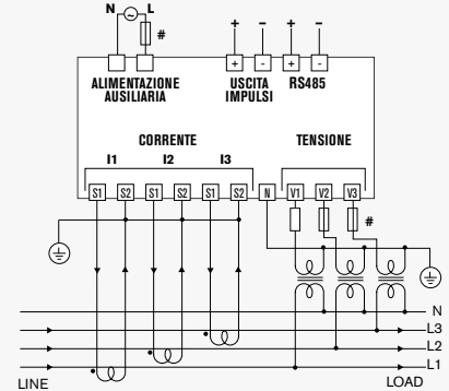
TRIFASE CON NEUTRO, 3 CT E 3 TRASFORMATORI DI TENSIONE
