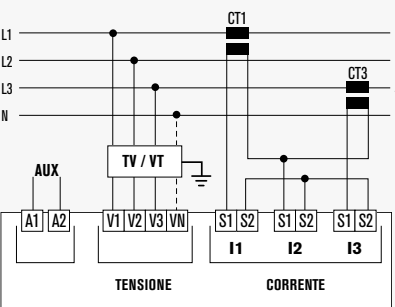
TRIFASE CON INSERZIONE ARON MEDIANTE TV Solo per la versione con TA interni
