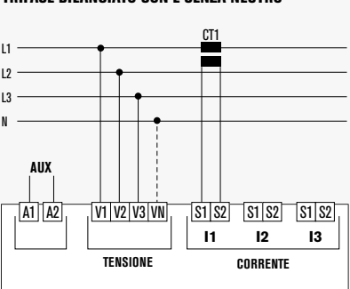
TRIFASE BILANCIATO CON E SENZA NEUTRO
