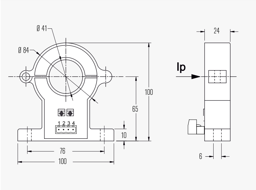
TTCA-41 - Dimensioni (mm)
