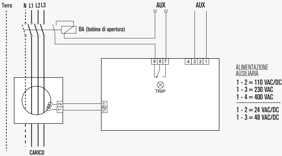
ELR-3E - Schema Elettrico
