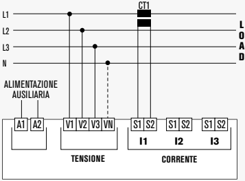
TRIFASE BILANCIATO CON E SENZA NEUTRO
