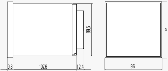
RDU-L - Dimensioni (mm)
