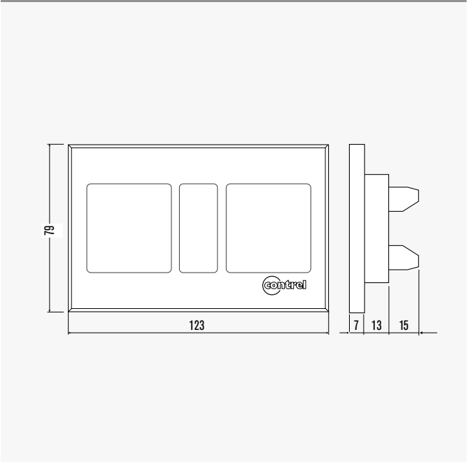
HPR-1 - Dimensioni (mm)
