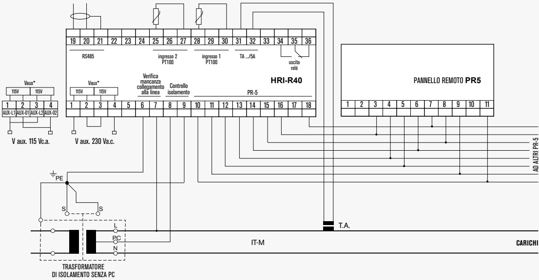
Con Trasformatore e CON presa centrale (pc)
