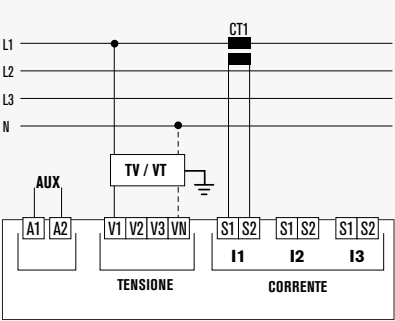
TRIFASE CON INSERZIONE MEDIANTE TV
