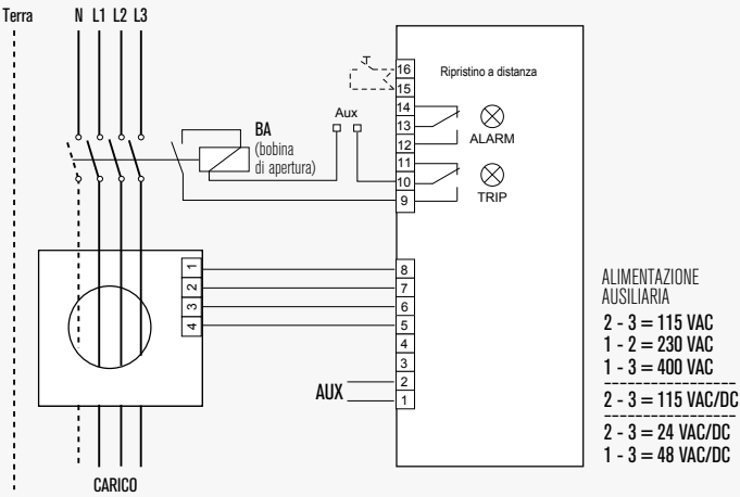
ELR-92 -Schema Elettrico
