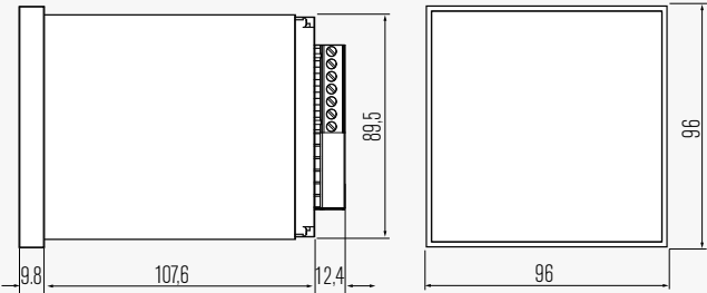
EMS-96 - Dimensioni (mm)
