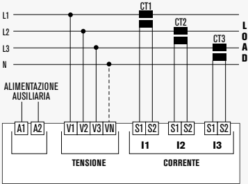
TRIFASE CON E SENZA NEUTRO
