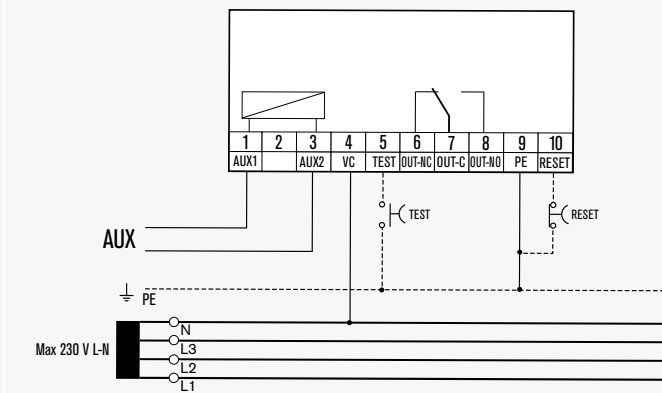
RI-F22 - Schema Elettrico
