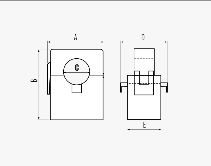
TTCAQ - Dimensioni (mm)
