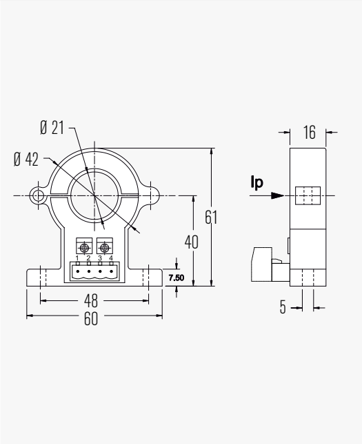
TTCA-21 - Dimensioni (mm)
