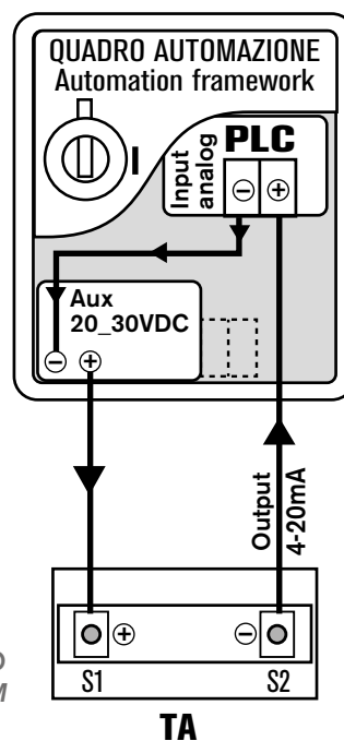
SCHEMA DI COLLEGAMENTO WIRING DIAGRAM
