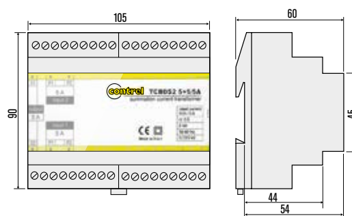
DIMENSIONI DIMENSIONS (mm)
