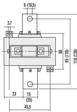
FISSAGGIO FIXING (mm)
