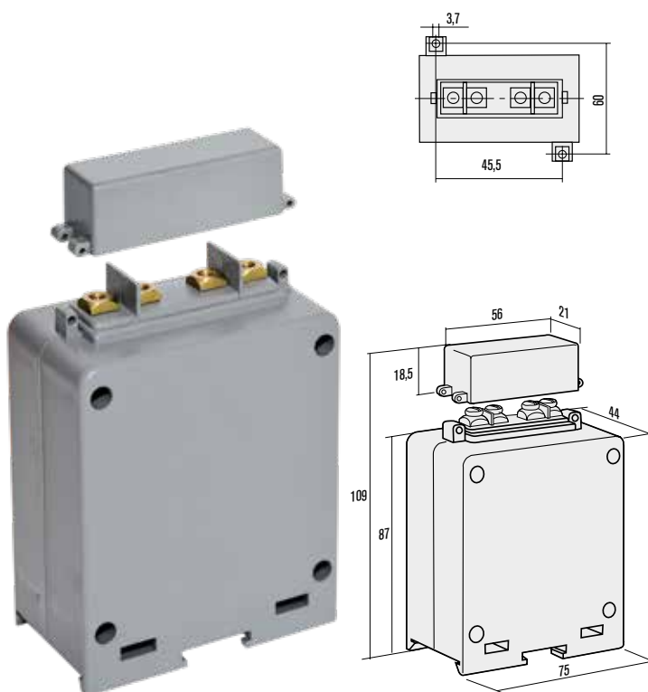
DIMENSIONI DIMENSIONS (mm)
