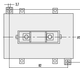
FISSAGGIO FIXING (mm)
