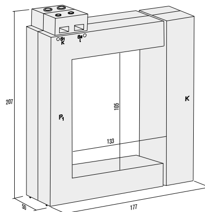
DIMENSIONI DIMENSIONS (mm)
