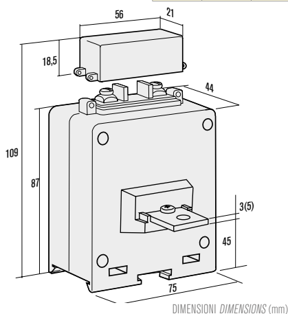
DIMENSIONI DIMENSIONS (mm)
