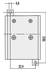
FISSAGGIO / FIXING (mm)
