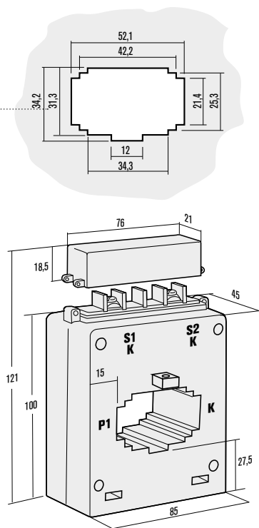
DIMENSIONI / DIMENSIONS (mm)
