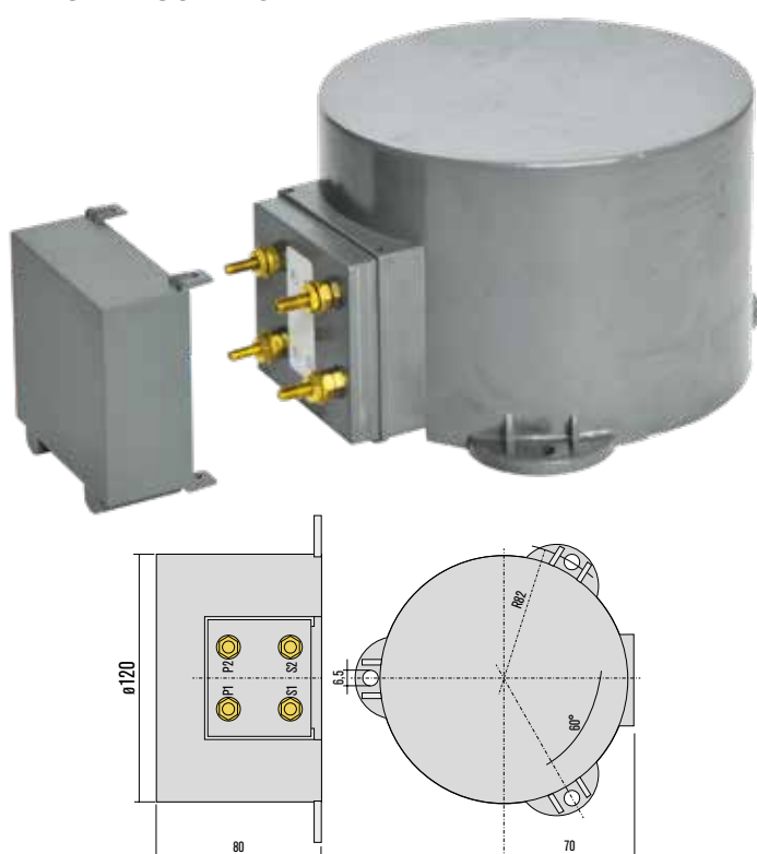
DIMENSIONI DIMENSIONS (mm)
