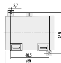
FISSAGGIO FIXING (mm)
