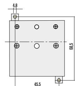
FISSAGGIO / FIXING (mm)
