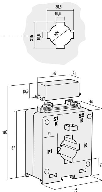
DIMENSIONI / DIMENSIONS (mm)
