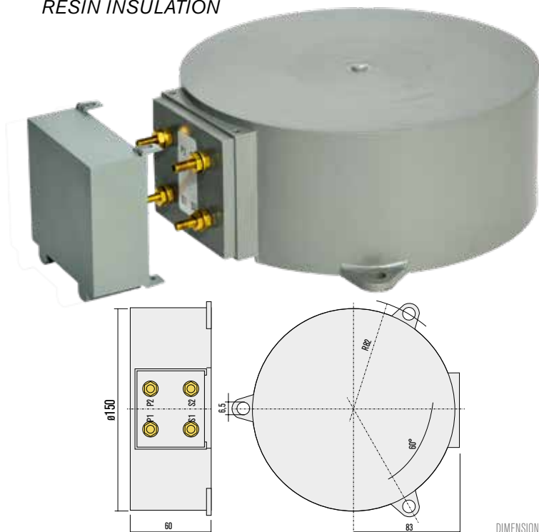
DIMENSIONI DIMENSIONS (mm)
