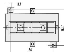
FISSAGGIO FIXING (mm)
