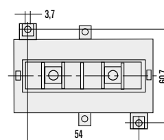
FISSAGGIO / FIXING (mm)
