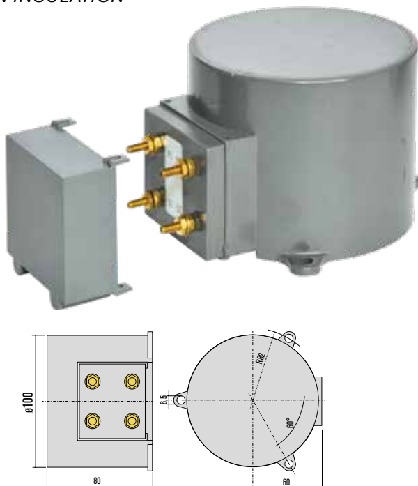
DIMENSIONI DIMENSIONS (mm)
